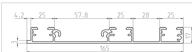
SBG 165 Selbstbauprofil Art.-Nr. 000472 Gewicht ca. 1700 g/m, Originalpackung 36 m
